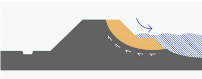
Dijk zakt weg aan rivierzijde (stabiliteit)
